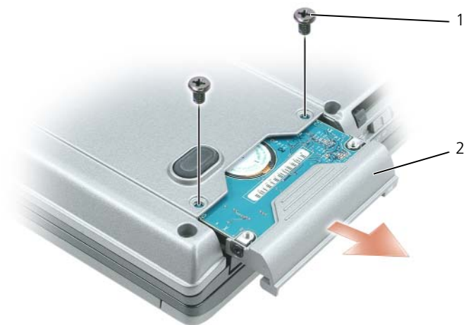
1 ネジ (2)
